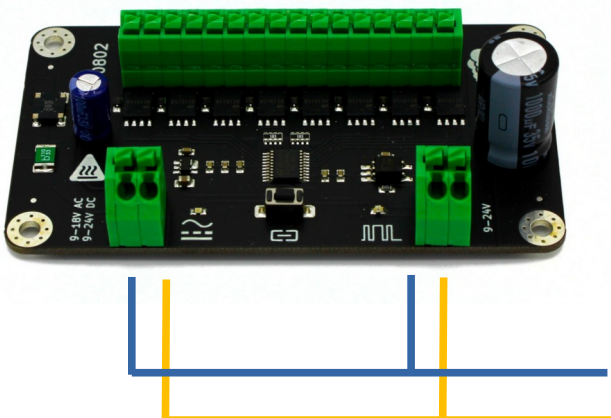
Programmiergleis
