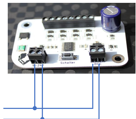
Programmiergleis
